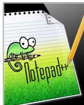
Notepad ++
